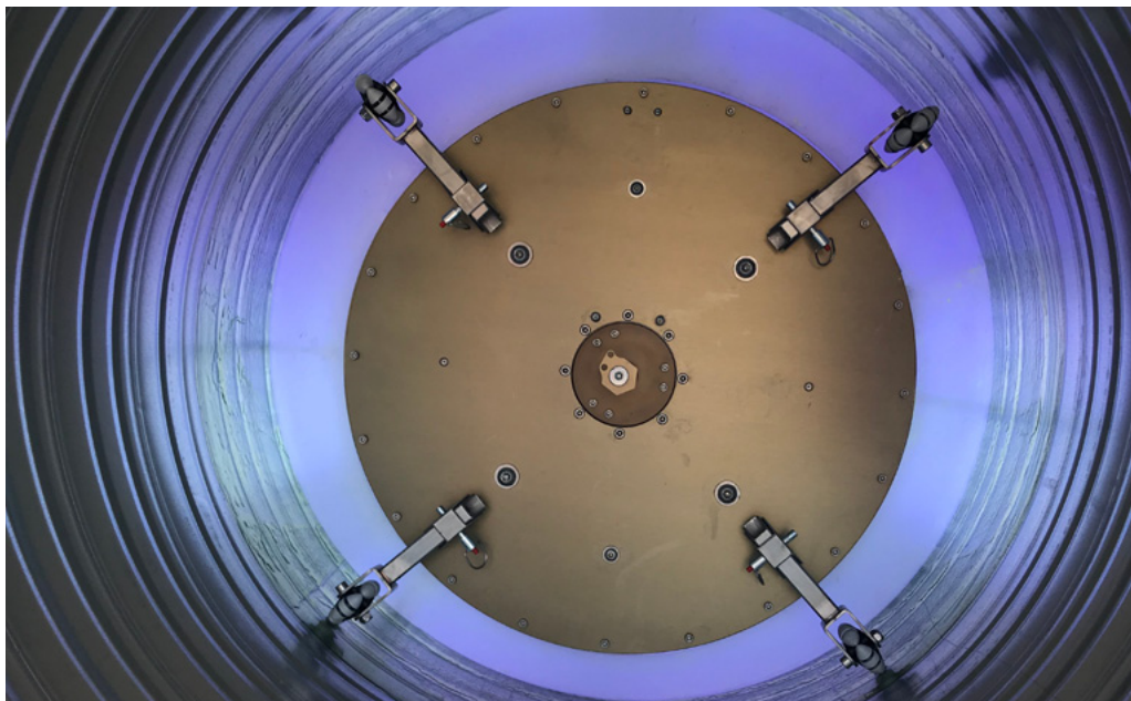
CIPP: Sistema a raggi ultravioletti - dettaglio di un treno luci
